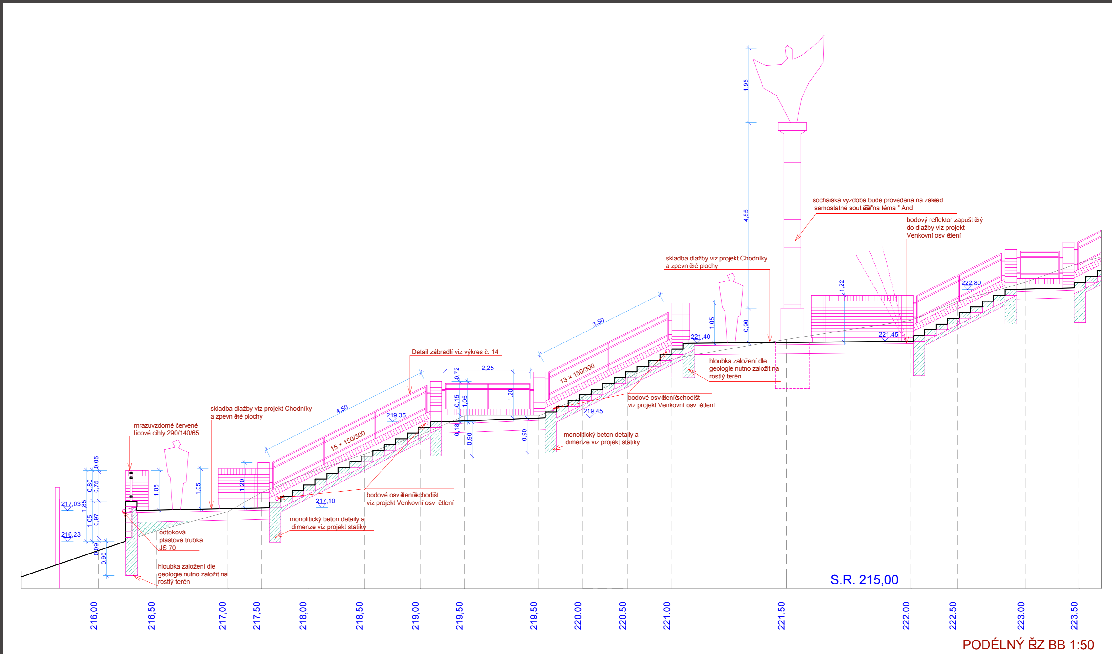
PODÉLNÝ ŘEZ BB 1:50
